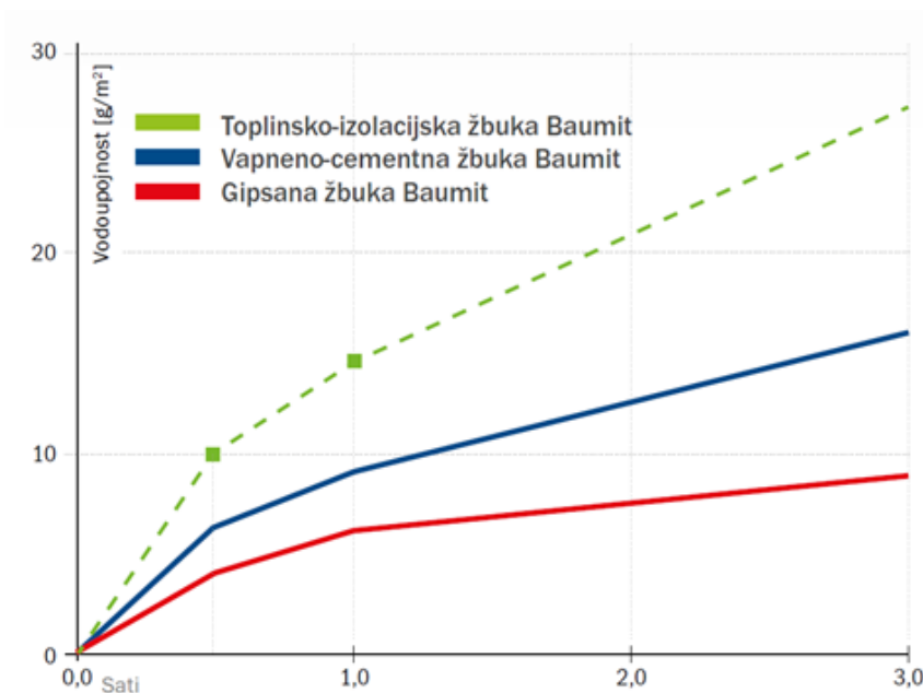
Dijagram apsorpcije vlage nakon 3 sata
